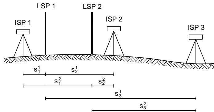
Abb. 2: Meßaufbau für die neu entwickelte Minimalkonfiguration
