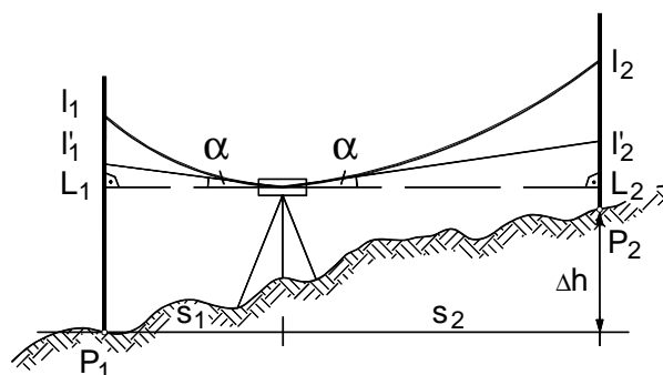
Abb. 1: Lattenablesungen im planaren Modell unter Einfluß von Restneigung und Refraktion
